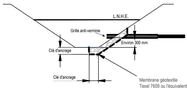
Coupe transversale
