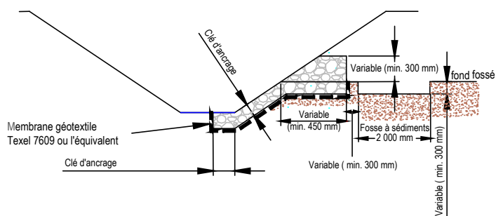
Coupe transversale
